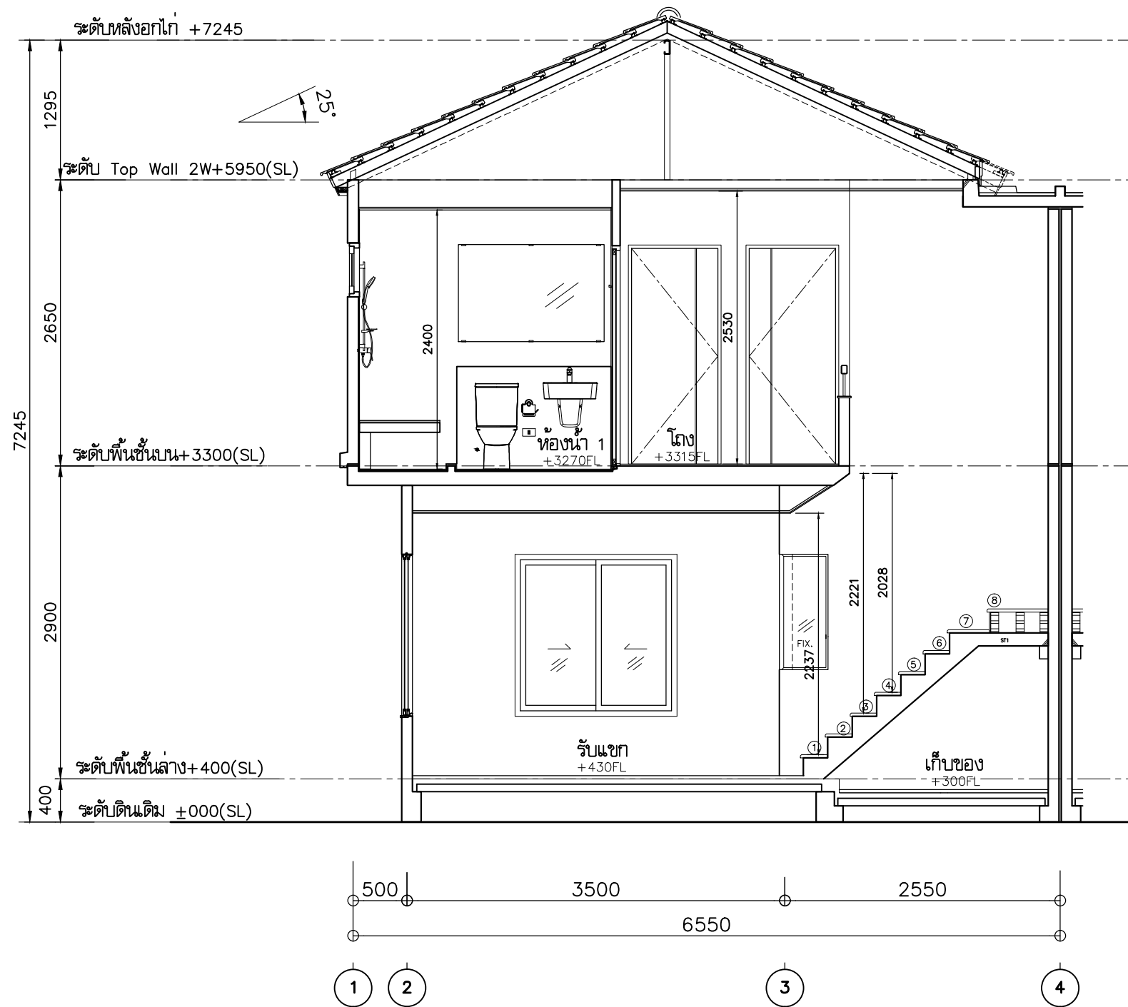
รูปตัด B - B 1 : 50
