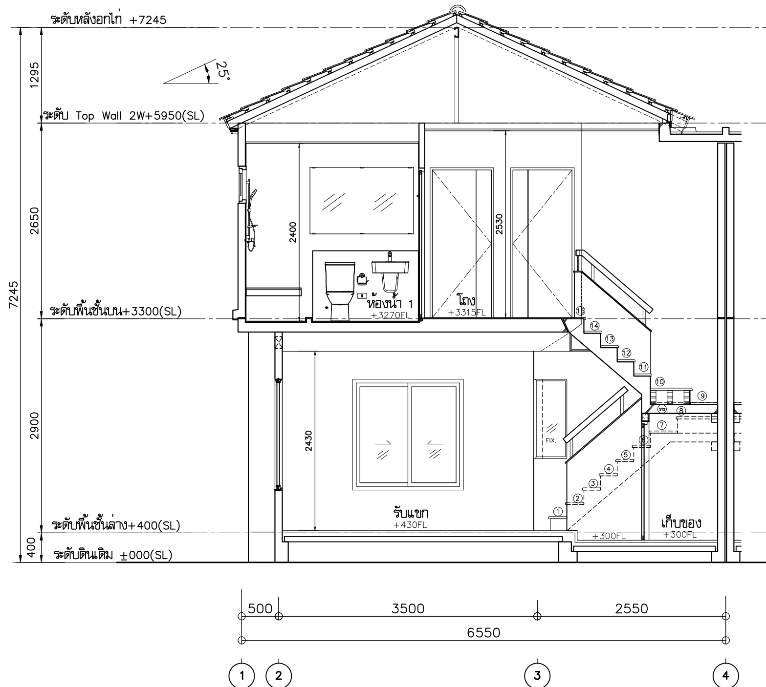
รูปตัด A - A 1 : 50
