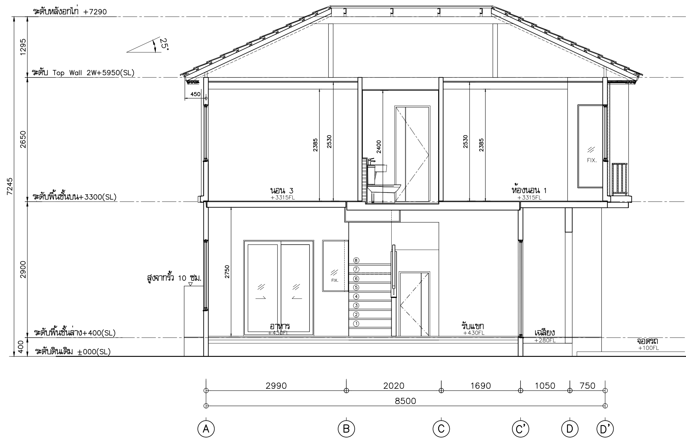
รูปตัด E - E 1 : 50
