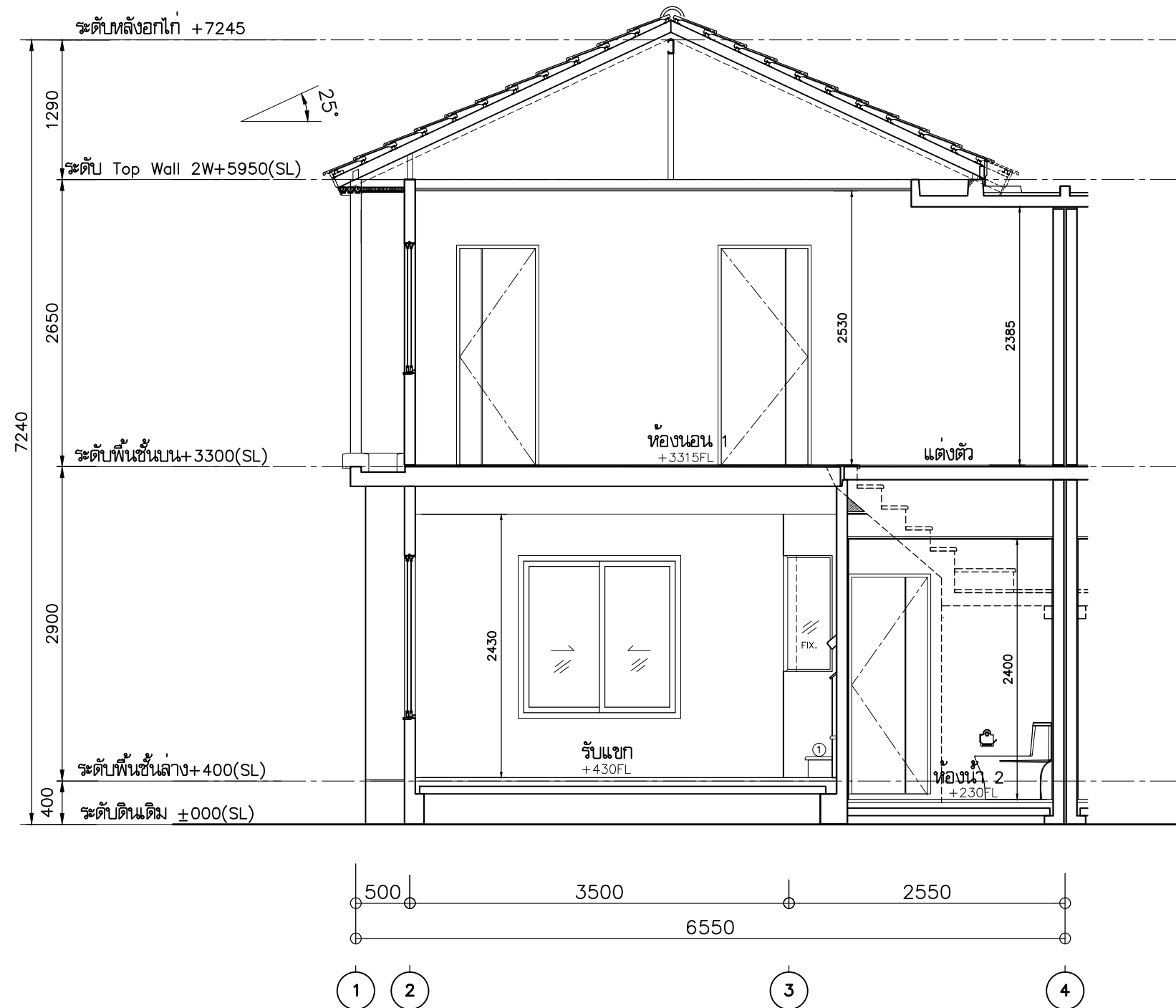
รูปตัด C - C 1 : 50
