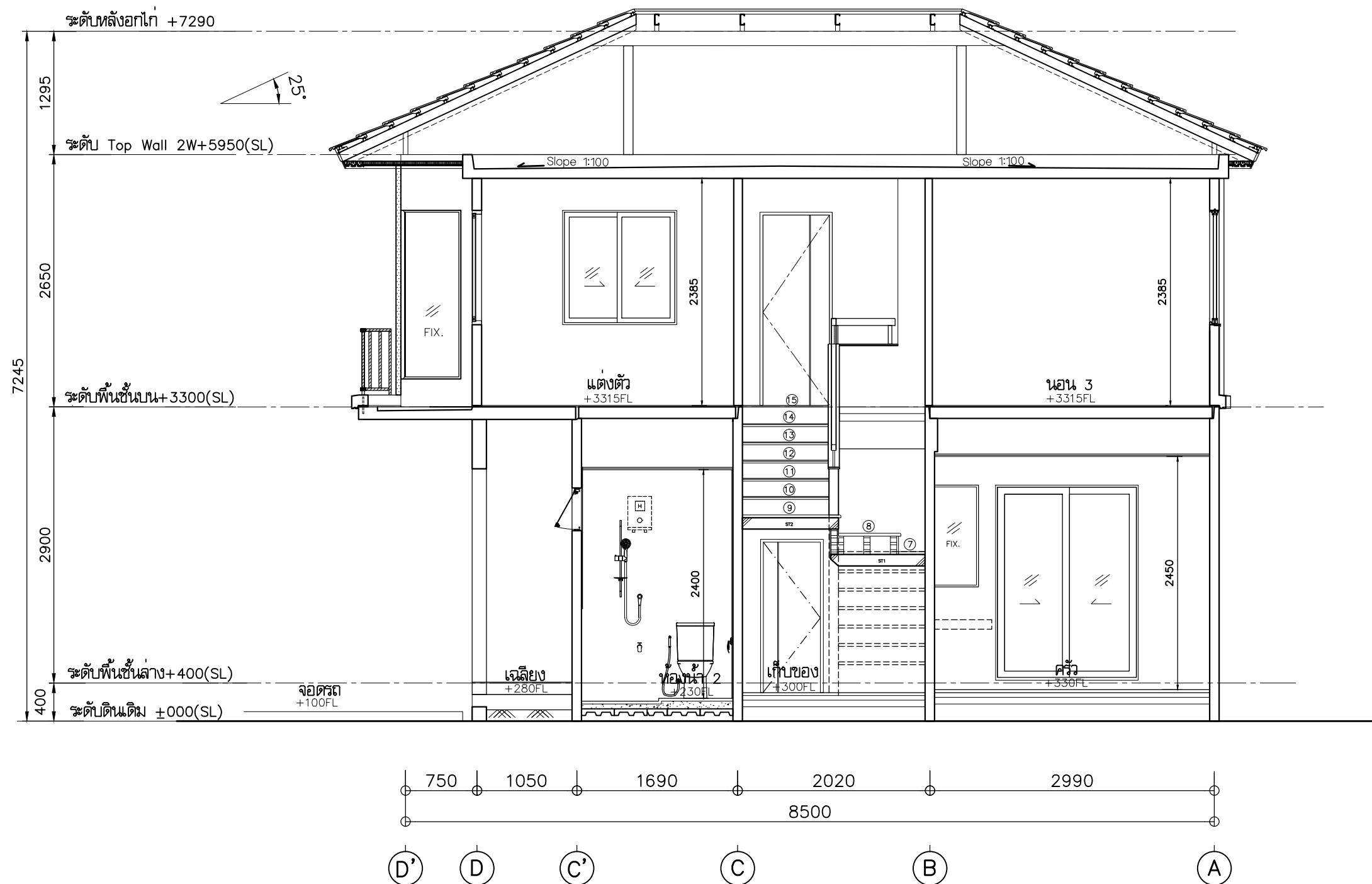
รูปตัด D - D 1 : 50
